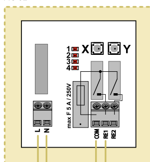
Alimentatore 230 V
